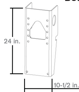
Hercules AJAX Style BUF1007-7327
